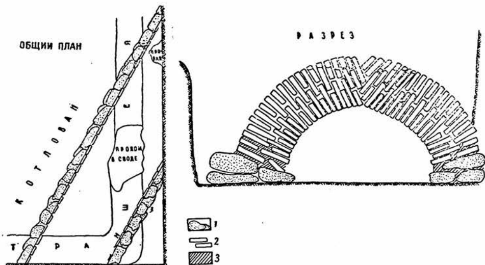
План канализационного сооружения XI—XII вв. в Ташкенте. Условные обозначения: 1—песчаник, 2—кирпич, 3—глина.
