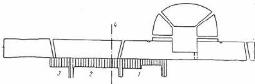
План башни в юго-восточной части городища Зартепа. Условные обозначения:
