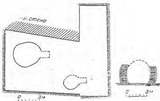
Рис. 1. Керамические печи с городища Эйлатан (план и разрез).
