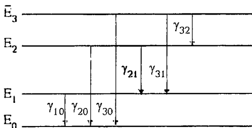
7-расм. {}_Z^AX^A ядронинг энергетик сатҳлари схемаси: E_0 – ядронинг асосий сатҳи; E_1 , E_2 , E_3 - уйғотилган ҳолатлар сатҳи.
