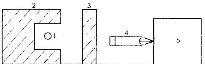
24-расм. Ўлчашига оид тажриба мосламаси
