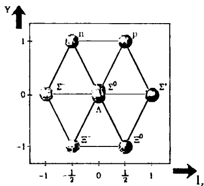
29-расм. Барион октети.
