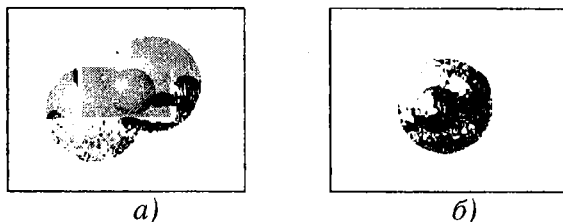
35-расм. Протон (а) ва нейтрон (б) ларнинг кварк ҳолати.
