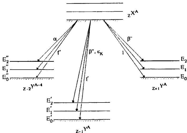
8-а расм. zX^A ядронинг емирилиш схемаси.
