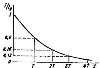
4-расм. Радиоактив емирилиш қонунининг график кўринишида тасвирланиши.
