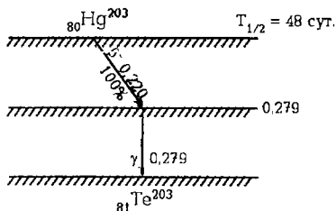
8-в расм. Баъзи радионуклидларнинг емирилиш схемалари. (β-, γ-нурланишларнинг энергияси МэВ ларда берилган.)
