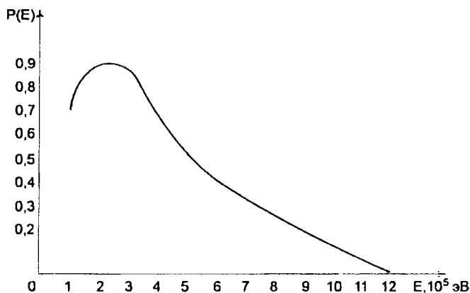
9-расм. Бета-зарраларнинг энергия спектри. ( \text{Te}^{40} )
