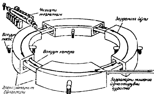
19-расм. Синхрофазотроннинг принципиал схемаси.
