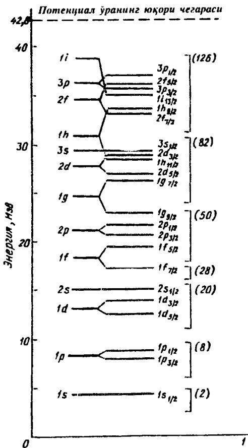
1-расм. Энергетик сатҳлар ва уларнинг қобикларга группаланиши.
