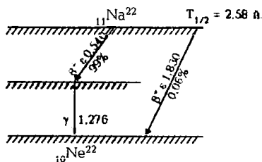
8-в расм. Баъзи радионуклидларнинг емирилиш схемалари. (β-, γ-нурланишларнинг энергияси МэВ ларда берилган.)
