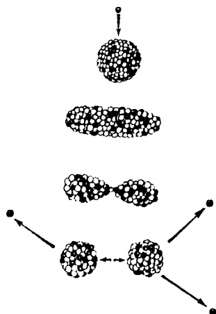
12-а расм. Ядронинг нейтрон таъсирида ядро бўлақларига ажралиб кетиш схемаси.
