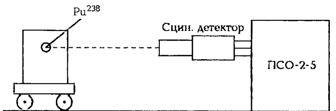
26-расм. Тажриба мосламалари.
