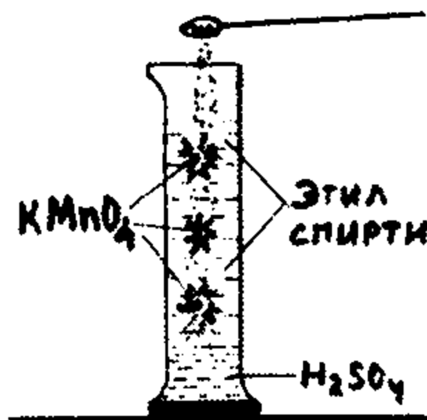
21-rasm. O'lchov silindrida mushakbozlik.
