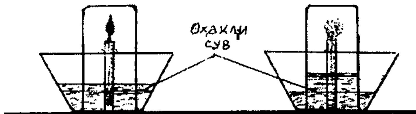
24-rasm. "Suv"ning yuqoriga ko'tarilishi.
