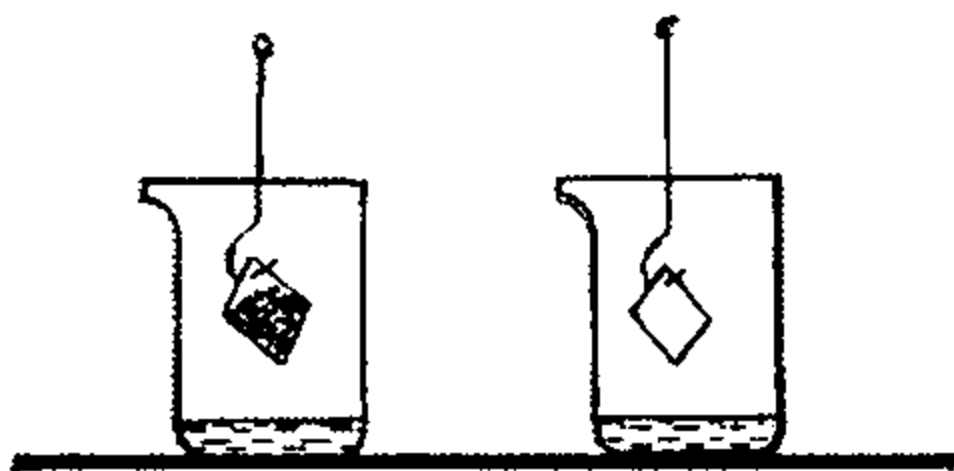
1-rasm. Rasmning paydo bo'lishi va yo'qolishi.
