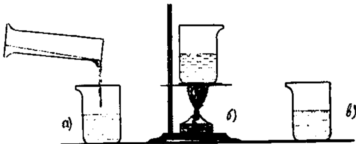
4-rasm. "Alkimoviy oltin" ning hosil bo'lishi.
