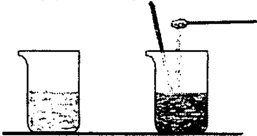
8-rasm. Ko'k rangli eritmaning olinishi.
