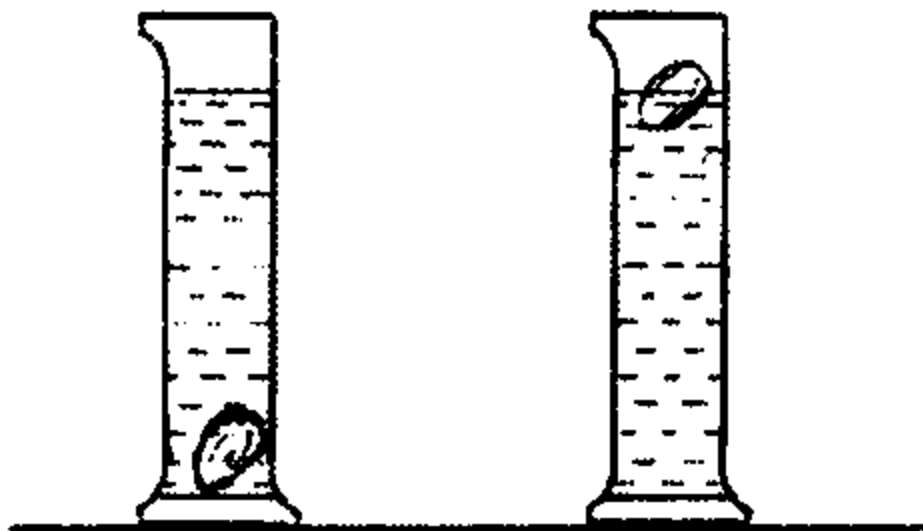
29-rasm. Tuximlarning cho‘kishi va cho‘kmasligi.
