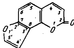
Фууро-2'-3', 7-8- кумарин, ангелицин
