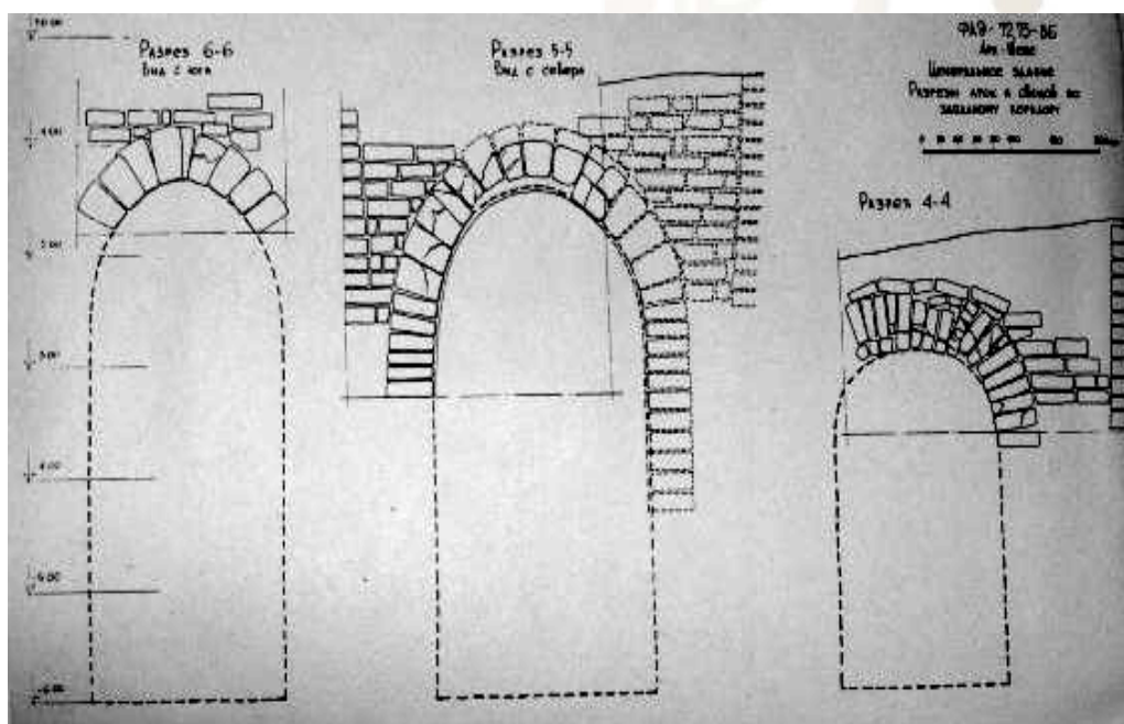
Аркасимон йулакларнинг кесими.
