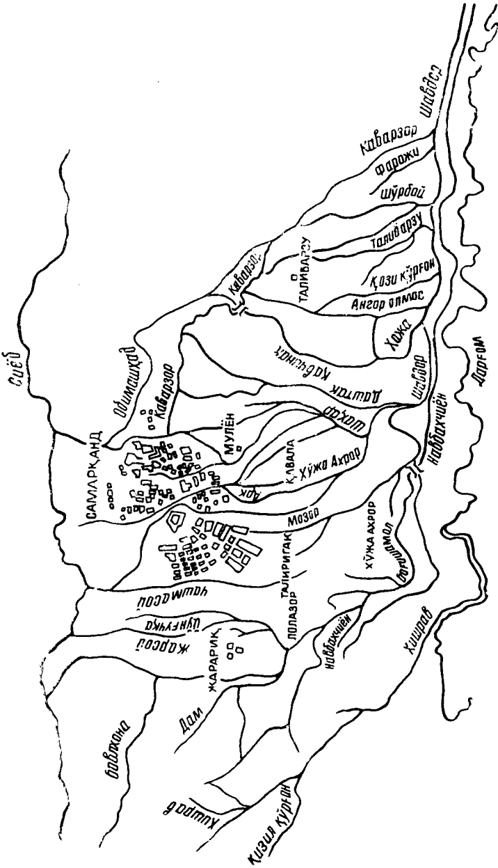
Илк ўрта асрларда Самарқанд ва унинг теварак-агрофн суториш системасининг схемаси.
