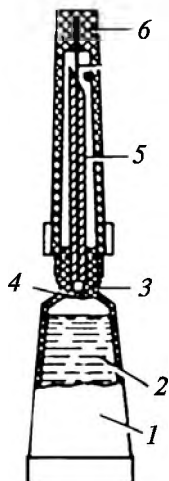
80-súwret. Shpric-tyubik: 1—antidot salınǵan plastmassalı tyubik; 2—antidot, 3—kanyula; 4—membrana; 5—iyne; 6—qaqpaqsha.
