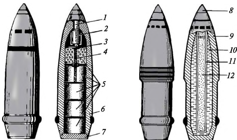
6-súwret. 115 mm li ximiyalıq artilleriya snaryadları: 1,8 — jarılıǵıshlar; 2 — porox zaryad; 3 — diafragma; 4 — tesilgen tütikshe; 5 — záhárlewshi zatlar shashkası; 6, 9 — korpus; 7 — snaryadnıń astıngı bólimi; 10 — záhárlewshi zat; 11 — jarıwshı zaryad ústingi stakanı; 12 — jarılıwshı zaryad.
