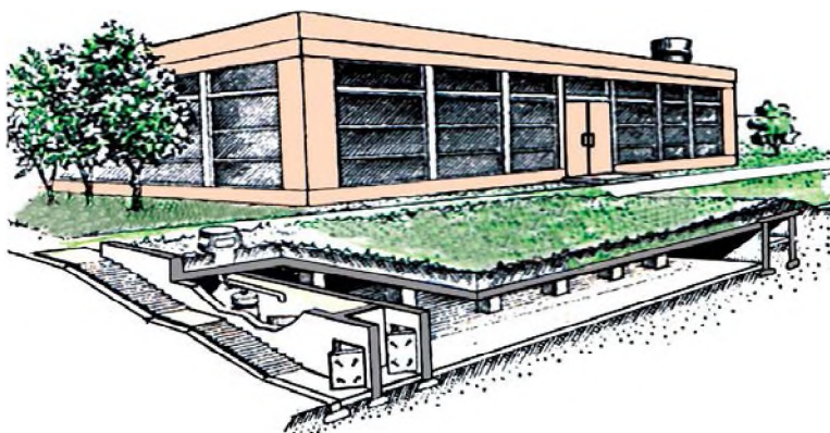
19-súwret. Óz aldına jaylasqan baspana.
