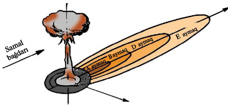
2-súwret. Yadro zaryadınıń jarılıwı nátiyjesinde payda bolǵan radioaktiv «iz».
