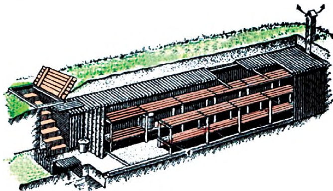
20-súwret. Radiaciyaǵa qarsı baspana.
