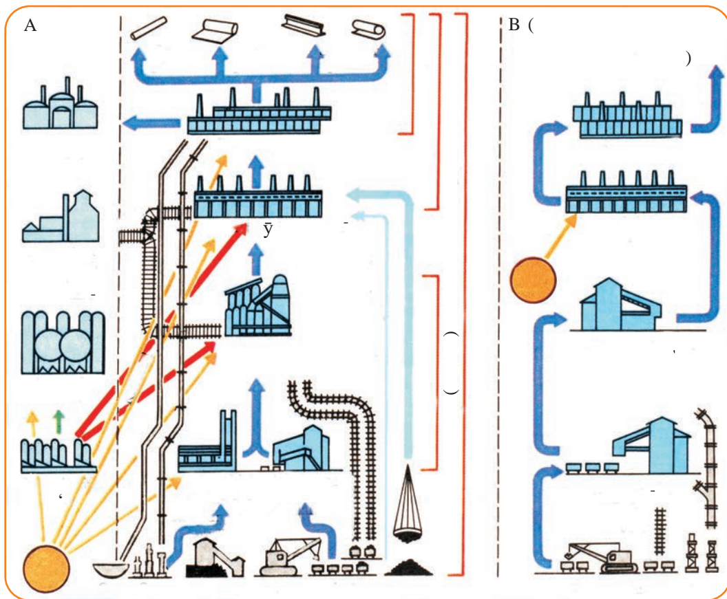
Расми 35. Схекаи сеҳҳои комбинати металлургӣ.
