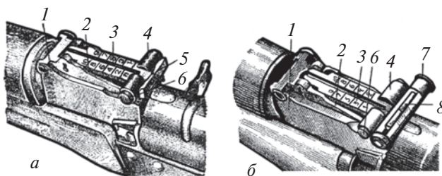
Расми 95. Ускунаи нишонгирӣ: а—барои автомат; б—барои пулемёт; 1—асоси ускуна; 2—рахҳои ускуна; 3—планка; 4—ҳалқаи ҳаракаткунанда; 5—чуқурчаи планкаи нишонгирӣ; 6—кашаки ҳалқаи ҳаракаткунанда; 7—тобдихандаи винти нишонча; 8—нишонча.
