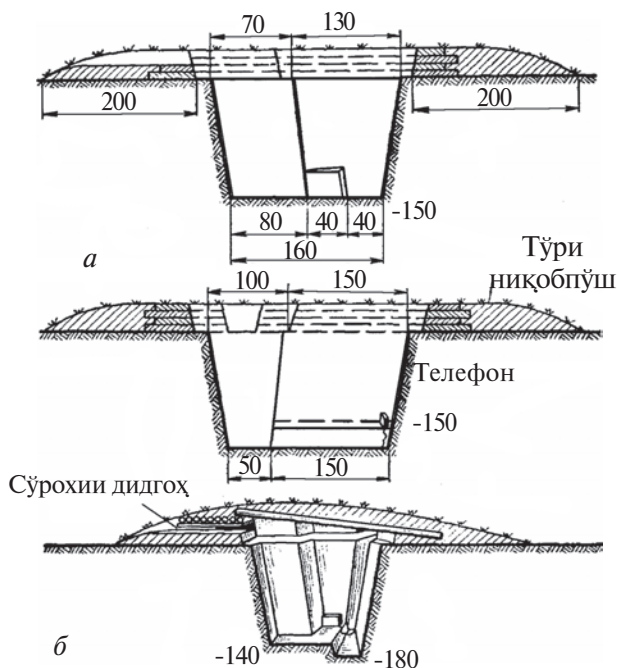
Расми 64. Пункти мушоҳида: a — хандақи кушод; б — хандақи болопўшида
