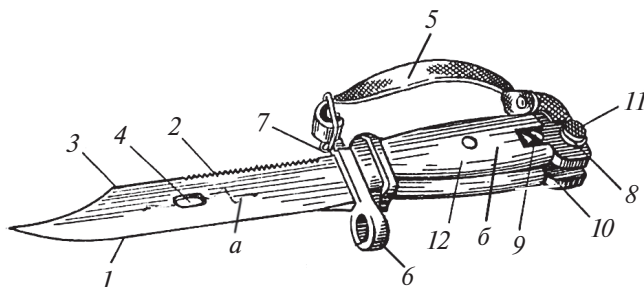
Расми 103. Найза-корд: а —теғ; б —даста; 1 —қирраи бурранда; 2 —арра; 3 —нўги чархшуда; 4 —сўрохи; 5 —камар; 6 —ҳалқа; 7 —чангак барои камар; 8 —қисми металии даста; 9 —винти пайвасти; 10 —буриш; 11 —кашиш; 12 —соп.
