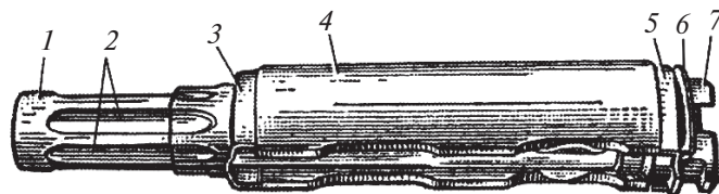
Расми 99. Трубкаи газ якҷоя бо ғилофи мил: 1—трубкаи газ; 2—қабурғаҳои самтбахш барои поршени газ; 3—пайваस्तкунандаи пеш; 4—ғилофи болои мил; 5—пайваस्तкунандаи ақиб; 6—тобдиҳанда; 7—пружинаи паҳн.
