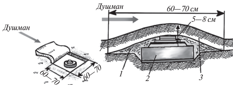
Расми 75. Гузоштани минаи зиддитанкӣ дар замини бо чим пӯшонидашуда: 1—бо хок пур кардан; 2—мина; 3—чими ниқобпӯш.
