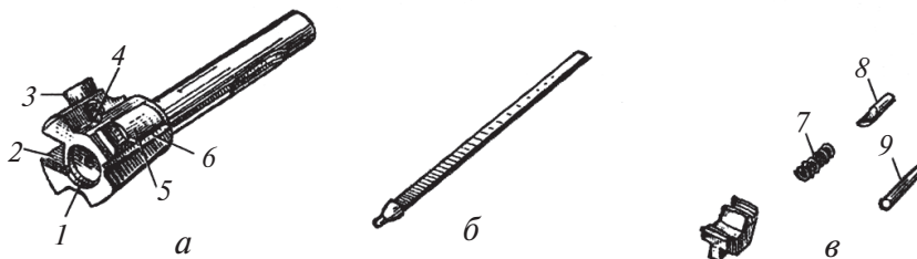
Расми 97. Затвор: а—асоси затвор; б—зарбадиҳанда; в—ҳаводиҳанда; 1—буриш барои гилза; 2—буриш барои ҳаводиҳанда; 3—пешбаранда; 4— чуқурча барои тири ҳаводиҳанда; 5—барҷастаи ҷанги; 6—буриш барои боздоранда ; 7—пружинаи ҳаводиҳанда; 8—тириҳаводиҳанда; 9—исканҷа.
