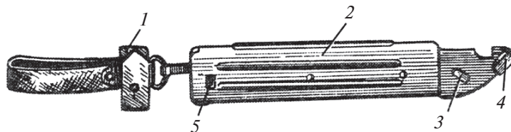
Расми 104. Қин: 1 —чангак, якҷоя бо камар ва карабин; 2 —ғилофи пластмасса; 3 —тири барҷаста; 4 —асос; 5 —пайвасткунандаи пружинаи паҳн.
