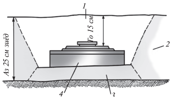
Расми 80. Гузоштани минаи зиддитанкӣ дар зимистон (барф): 1—барфи ниқоби; 2—барф; 3—барфи зичшуда; 4—мина.
