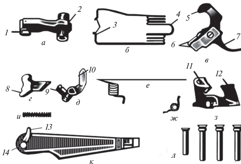
Расми 100. Қисмҳои механизми зарбадиҳанда: а—зарбадиҳанда; б—пружинаи ҷангӣ; в—чангак; з—шепталои якка тирандозӣ; д—автозарбадиҳанда; е—пружинаи автозарбадиҳанда; ж—гузаронанда; з—тир ва пружинаҳои шептало; и—хомӯшкунандаи ҳаракати зарбадиҳанда; к—пружинаи хомӯшкунанда; л—тири кубуршакл; 1—сатҳи ҷангӣ; 2—сатҳи автозарбадиҳанда; 3—нўгҳои қатшуда; 4—часпак; 5—тобдиҳандаи қач; 6—тобдиҳандаи росткунҷа; 7—думча; 8—парча; 9—шептало; 10—тирак; 11—зашелка; 12—тобдиҳандаи пеш; 13—худуди гузаронанда; 14—саффа.
