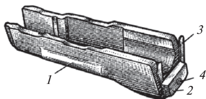
Расми 101. Гилофи зери мил (даста): 1—қой барои ангушт; 2—тобдиҳанда; 3—пружинаи паҳн; 4—шикоф барои шимпол.
