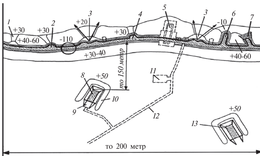
Расми 73. Сексияи хандақ: 1—майдони ҷанг; 2—гузаргоҳҳо ба паҳлӯ; 3—ҷойи пулемётҳо; 4—ҷойи оташфишони; 5—истеҳкоми болопӯшида; 6—ҷойи гранатомёт; 7—майдони ҷангии болопӯшида; 8—ҷой барои БМП дар позитсияи асосии оташфишони; 9—аппарел; 10—тӯдаи хок; 11—ҷойи зарурат; 12—роҳҳои алоқа; 13—ҷой барои БМП дар вазъияти аз захира оташ кушодан.
