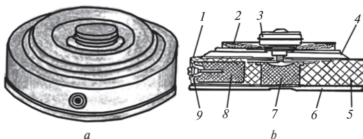
Расми 74. Намуди минаи зиддитанкӣ ТМ-57 бо тарканди MVZ-57: а—намуди умумӣ дар ҳолати нақлиётӣ; б—намуди ҳолати ҷангии мина дар бурриш: 1—корпус; 2—сипарча; 3—тарканди MVZ-57; 4—диафрагма (парда монеа); 5—заряд; 6—зер; 7—детонатори марказӣ; 8—детонатори паҳлӯ; 9—сарпӯш.
