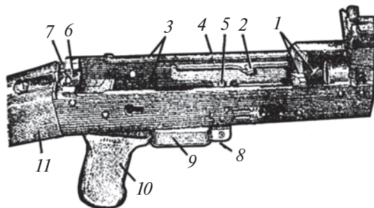
Расми 93. Қуттии мил: 1—буришҳо; 2—бозгардон; 3—барҷастаҳо; 4—барҷастаи самтноққунанда; 5—пайвасткунанда; 6—фосилаи яксара; 7—фосилаи буришӣ; 8—исканҷаи магазин; 9—ҳалқаи теладиханда; 10—дастаи пистолет; 11—қундоқ
