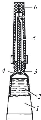
80-nji surat. Şpris-týubik: 1 — antidot salnan plastmassaly týubik; 2 — antidot; 3 — kanýula; 4 — membrana; 5 — iňňe; 6 — galpak.
