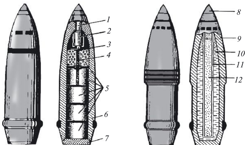
6-njy surat. 115 mm-li himiki artilleriýa snaryadlary: 1, 8 — partladyjylar; 2 — poroh zarýady; 3 — diafragma; 4 — deşilen näý; 5 — zäherleýji maddalaryň şaşkasy; 6, 9 — korpus; 7 — snaryadyň aşaky bölegi; 10 — zäherleýji madda; 11 — partladyjy zarýad üstki stakany; 12 — partladyjy zarýad.
