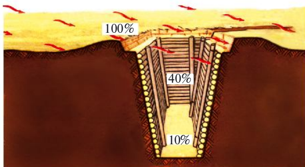
3-nji surat. Hendegiň radioaktiw şöhleleri peseldiji aýratynlygy.
