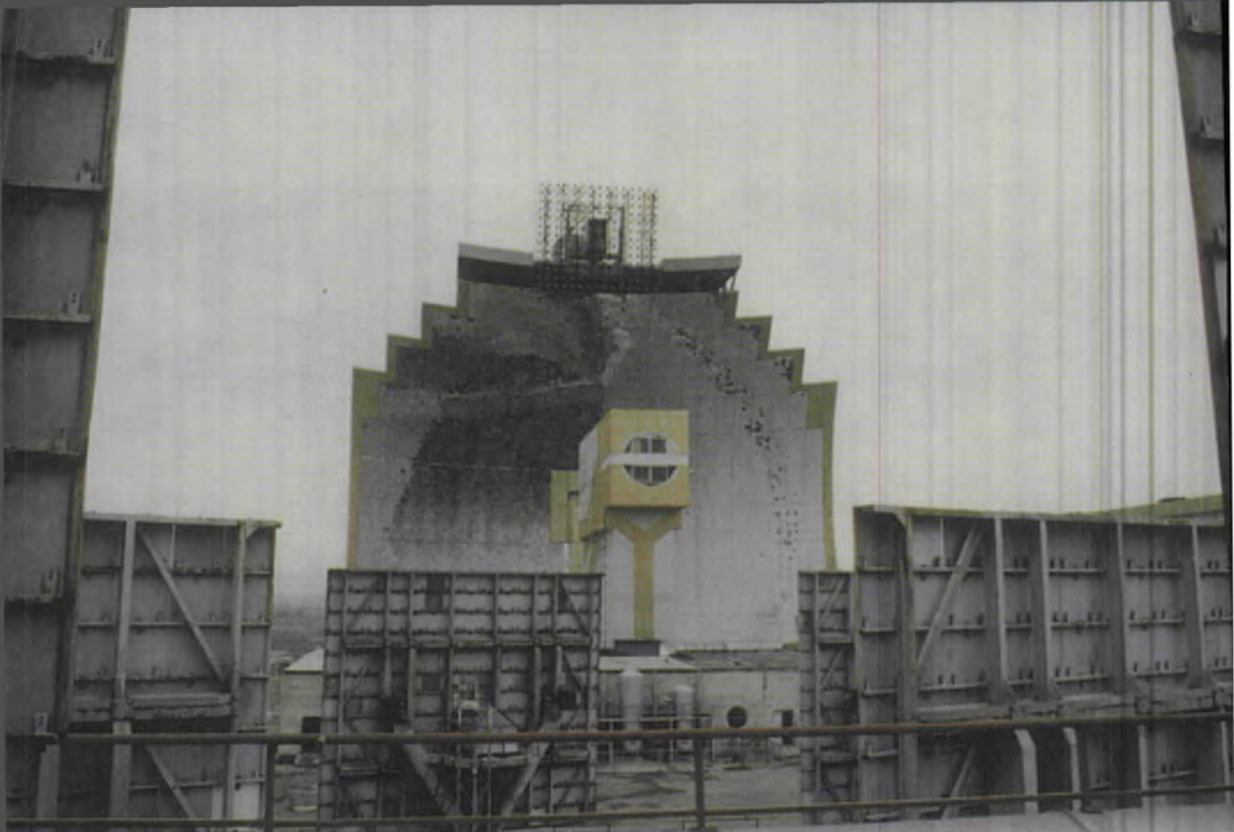
Ўзбекистон Республикаси Фанлар академияси "Физика-Қуёш" материалшунослик институтининг катта қуёш печи.
