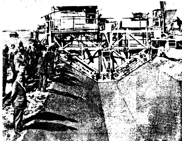
Бетонирование канала.
