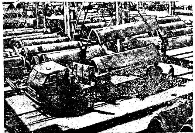
Оросительные лотки, изготавливаемые на Каршинском заводе железобетонных изделий.
