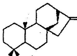
Ent-kauren
