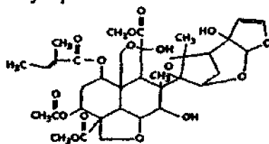
Azadiraxtin
