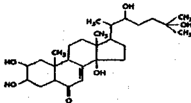
\alpha -Ekdison
