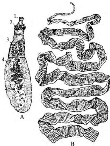
61-rasm. Har xil tasmasimon chuvalchaglar:
