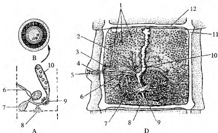
58-rasm. Qoramol tasmasimon chuvalchangining rivojlanish sikli. A – urg'ochilik jinsiy sistemasining tuzilishi sxemasi. B – onkosferali tuxum, D – qoramol tasmasimoni germafrodit bo'g'imi.
