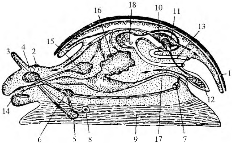
102-rasm. Qorinoyoqli mollyuskalarning tuzilishi sxemasi. 1 – chigʻanoq, 2 – koʻz, 3 – paypaslagich, 4 – bosh nerv gangliysi, 5 – oyoq nerv gangliysi, 6 – plevral gangliy, 7 – visceral gangliy, 8 – statotsist, 9 – oyoq, 10 – yurak, 11 – yurakoldi xaltasi boʻshligʻi, 12 – jabralar, 13 – ayirish organlari, 14 – qirgʻich, 15 – soʻlak bezi, 16 – jigar, 17 – oʻrta ichak, 18 – jinsiy bez.
