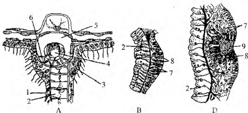
37-rasm. Gidromeduzalarning sezgi organlari.
