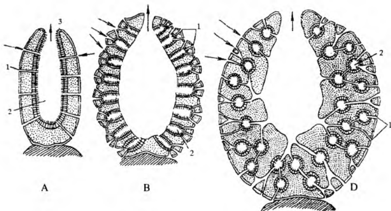
27-rasm. G'ovoktanlilarning tuzilish tiplari.
