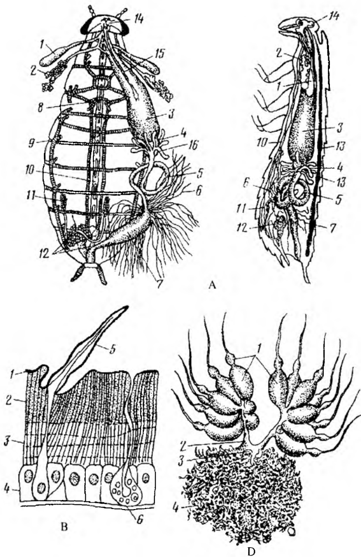
156-rasm. Qora suvarakning tuzilishi. A – ichki tuzilishi orqa va yondan ko'rinishi: 1 – so'lak bezi rezervuari, 2 – so'lak bezi, 3 – jig'ildon, 4 – muskulli oshqozon, 5 – o'rta ichak, 6 – malpigi naychalari, 7 – orqa ichak, 8, 9 – traxeya, 10 – qorin nerv zanjiri, 11 – urug'don, 12 – jinsiy bezlar, 13 – yurak, 14 – bosh-miya, 15 – simpatik nerv sistemasi, 16 – orqa ichakning pilorik (ko'r) o'simtalari; B – kutikulasining tuzilishi: 1 – epikutikula, 2 – ekzokutikula, 3 – endokutikula, 4 – gipoderma, 5 – qil, 6 – teri bezi; D – urg'ochilik jinsiy organi: 1 – tuxumdon naylari, 2 – tuxum yo'li, 3 – urug' qabul qilgich, 4 – bezlar.
