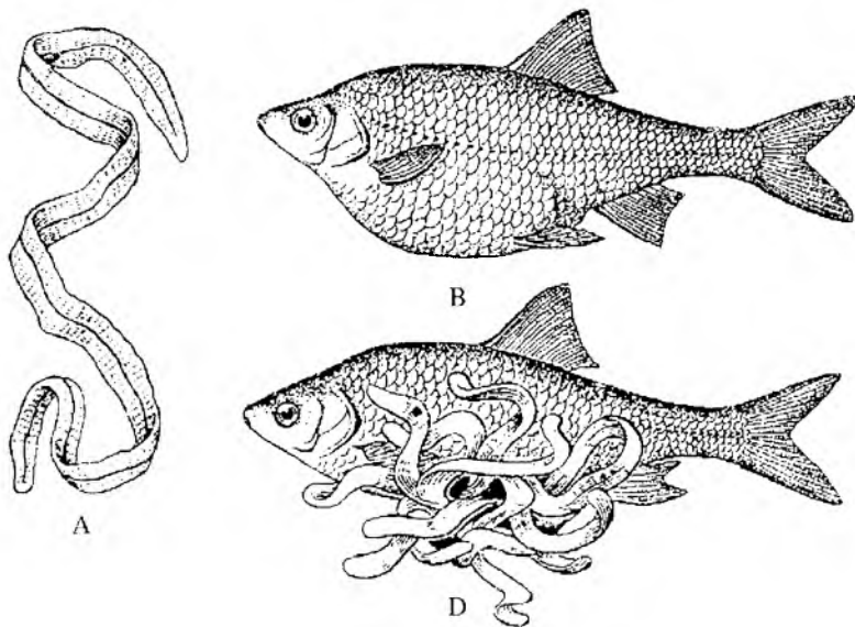
62-rasm. Tasmason chuvalchang Ligula.
