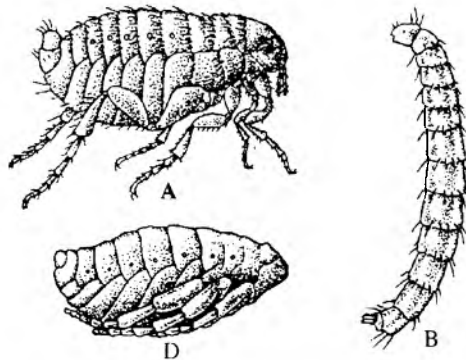
193-rasm. Odam burgasi. A – imago. B – lichinka. D – g'umbak.
