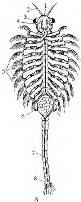
127-Artemiya jabraoyoqlisi Artemis salina . A – umumiy koʻrinishi. B – erkagining boshi: 1 – nauplius koʻz. 2 – antennulla. 3 – fasetkali koʻz. 4 – antenna. 5 – koʻkrak oyogʻi. 6 – tuxum xaltasi. 7 – qorin. 8 – ayri.
