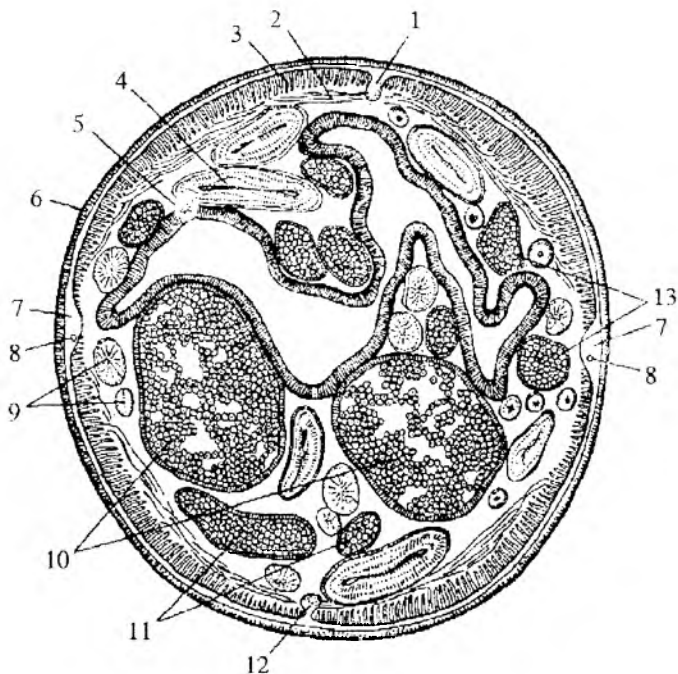
65-rasm. Urg'ochi askaridaning ko'ndalang kesmasi.
