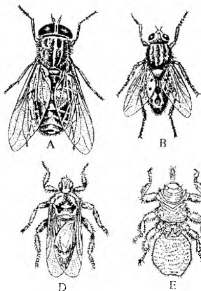
195-rasm. Kalta mo'ylov ikkiqanotlilar. A – so'na. B – volfart pashshasi. D – qonxo'r it pashshasi. E – qonxo'r qo'y pashshasi.
