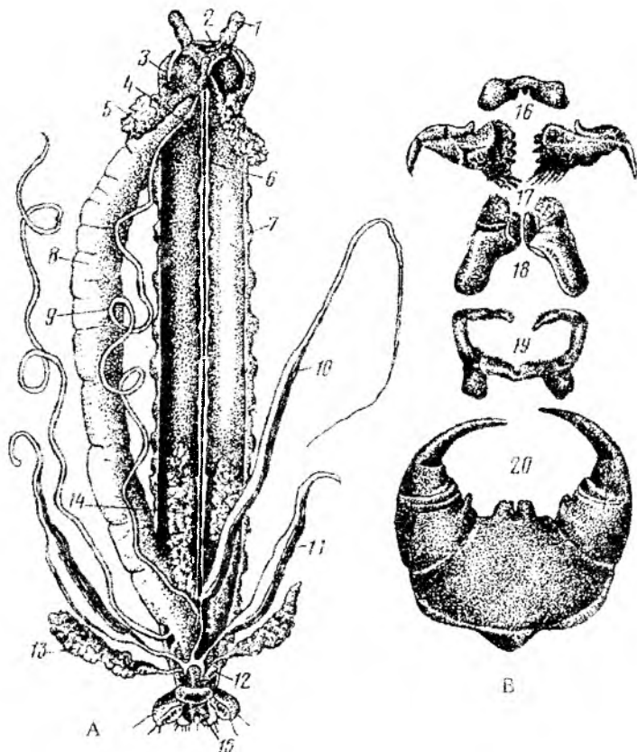
145-rasm. Ko'poyoqlilarning tuzilishi. A -- ichki tuzilishi. B -- og'iz organlari: 1 -- mo'ylov, 2 -- halqumusti gangliyi, 3 -- zahar bezli jag'oyoq, 4 -- qizilo'ngach, 5 -- so'lak bezi. 6 -- qorin nerv zanjiri, 7 -- oyoq, 8 -- o'rta ichak, 9 -- malpigi naychalari. 10 -- urug'don, 11 -- urug' pufagi 12 -- urug' yo'li, 13 -- keyingi bez.
