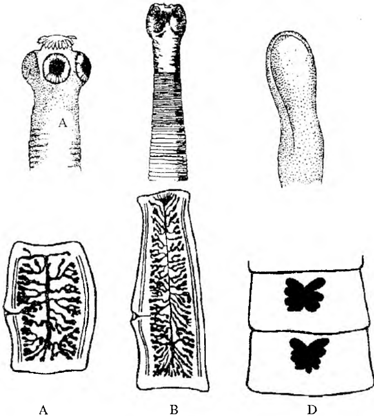
57-rasm. Tasmasimon chualchanglar so'rg'ichlari va proglotidlari. A – cho'chqa tasmasimoni. B – qoramol tasmasimoni. D – keng tasmasimon.
