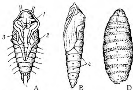
167-rasm. Hasharotlar g'umbaklari.
