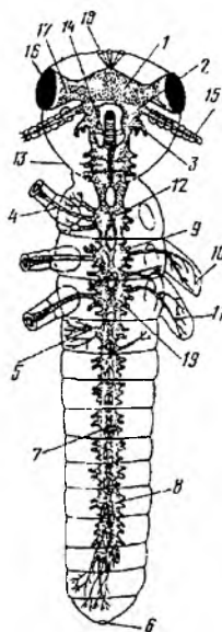
157-rasm. Hasharotlar markaziy nerv sistemasining tuzilishi.
