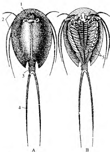
128-rasm. Qalqondor Triops cancriformis .
