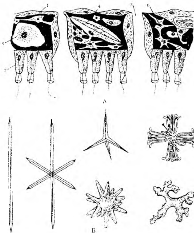
28-rasm. G'ovaktanlilarining tuzilishi.
