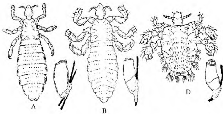
186-rasm. Odam bitlari va ularning sirkalari. A – bosh biti. B – kiyim biti. D – chov biti.
