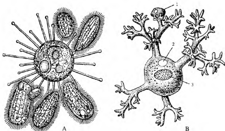
25-rasm. So‘ruvchi infuzoriyalalar.
