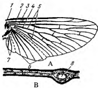
153-rasm. Hasharotlar qanotining tuzilishi.
