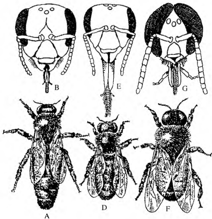
198-rasm. Asalari. A, B – urg‘ochi ari va uning boshi. D, E – ishchi ari va uning boshi. F, F – erkak ari va uning boshi.
