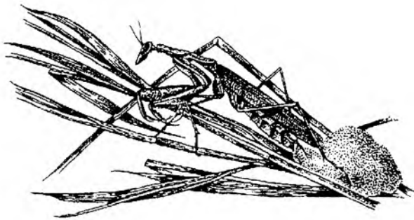
183-rasm. Oddiy beshiktebratar Mantis religiosa (qornining keyingi qismidan ajralib chiqayotgan ko'pikdan tuxumaxalta - ooteka hosil bo'ladi).
