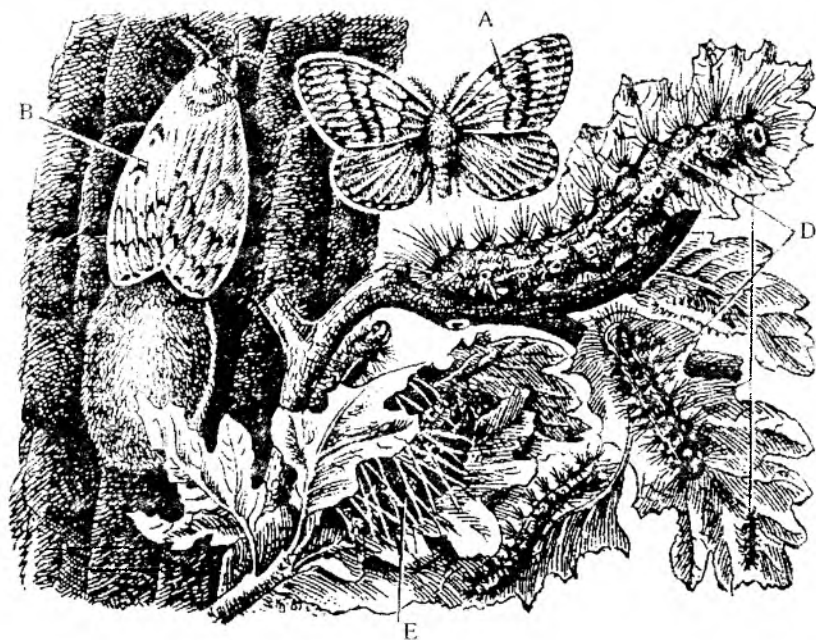
192-rasm. Juftsiz ipak qurti ( Ocneria dispar ). A – erkagi. B – tuxum qo'yayotgan urg'ochisi. D – har xil yoshdagi qurtlar. E – pilla ichidagi g'umbagi.
