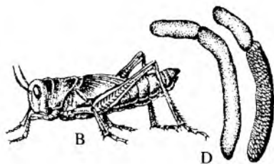
180-rasm. Osiyo chigirtkasi. A – imago (tuxum qo'yayotgan urg'ochisi va erkagi). B – lichinka. D – xumchalari.
