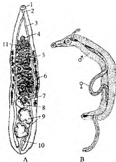
55-rasm. Odamda parazitlik qiluvchi so'rg'ichlilar.
