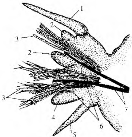
79-rasm. Nereis parapodiyasi.
