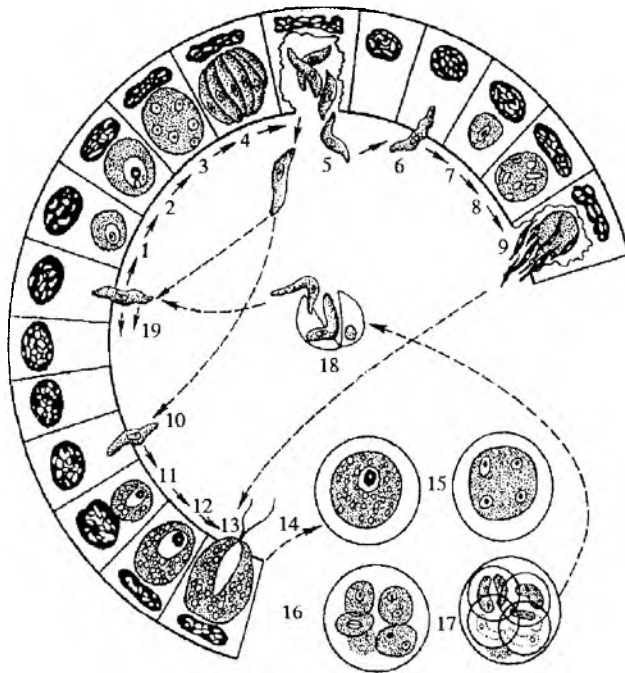
14-rasm. Koksidiyalar hayot sikli.
