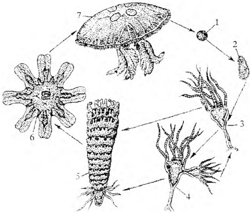
41-rasm. Sifoid meduzalarning rivojlanishi.
