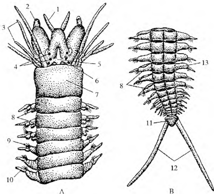
78-rasm. Nereising oldingi (A) va keyingi (B) tomoni.
