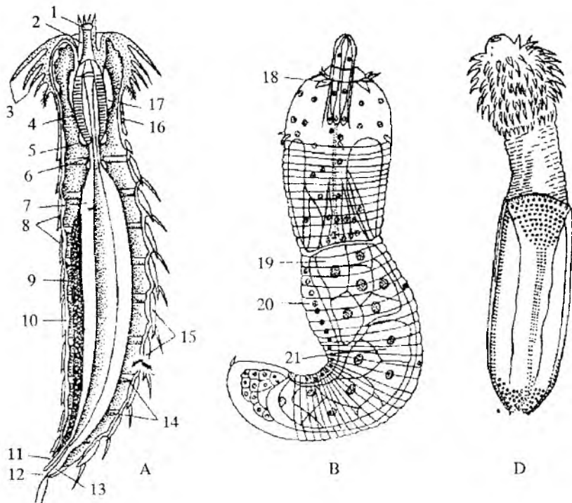
73-rasm. Kinorinxlar. A – kinorinxning tuzilishi sxemasi. B – qilchugalchang lichinkasi. D – priapulid lichinkasi: 1 – ogʻiz, 2 – ogʻiz boʻrtigʻi, 3 – bosh pixlari, 4 – halqum, 5 – orqa bezlari, 6 – qizil oʻngach, 7 – oʻrta ichak, 8 – qorin plastinkasi, 9 – jinsiy bez, 10 – qorin nervi, 11 – jinsiy teshik, 12 – anal teshik, 13 – orqa ichak, 14 – dorzo-ventral muskullar, 15 – orqa plastinkalar, 16 – boʻyin plastinkalari, 17 – halqumoldi nerv halqasi, 18 – ilmoqlar, 19 – halqum bezlari, 20 – qorin nerv stvoli boshlangʻichi, 21 – ichak.
