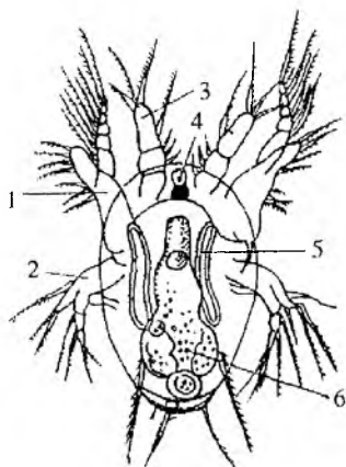
123-rasm. Qisqichbaqasimonlarning nauplius lichinkasi.
