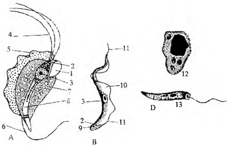
11-rasm. Parazit xivchinlari.
