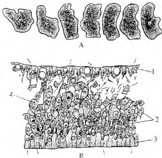
26-rasm. Trixoplaks. A – siljib harakatlanayotganida tana shaklining o‘zgarishi. B – kundalang kesimi: 1 – orqa epiteliysi. 2 – o‘rta qavatning mezenxima hujayralari. 3 – qorin epiteliysi. 4 – mezenxima hujayrasidagi hazim vakuolasi.
