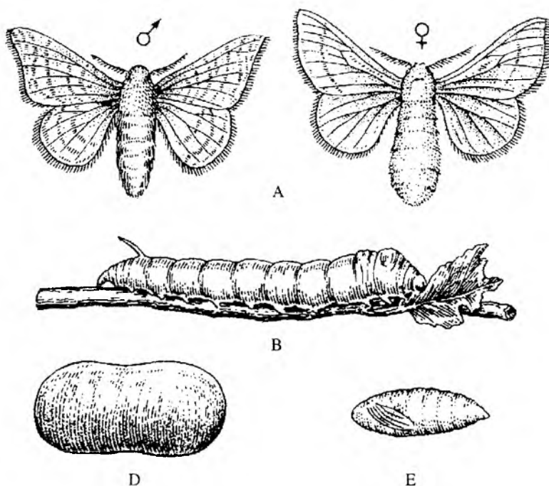
165-rasm. Tut ipak qurtining to‘liq metamorfoz orqali rivojlanishi. A – kapalak. B – qurt. D – pilla. E – pilladan chiqarib olingan g‘umbak.
