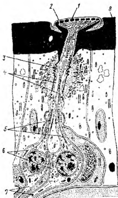
160-rasm. Hasharotlar hid bilish sensillarining tuzilishi.
