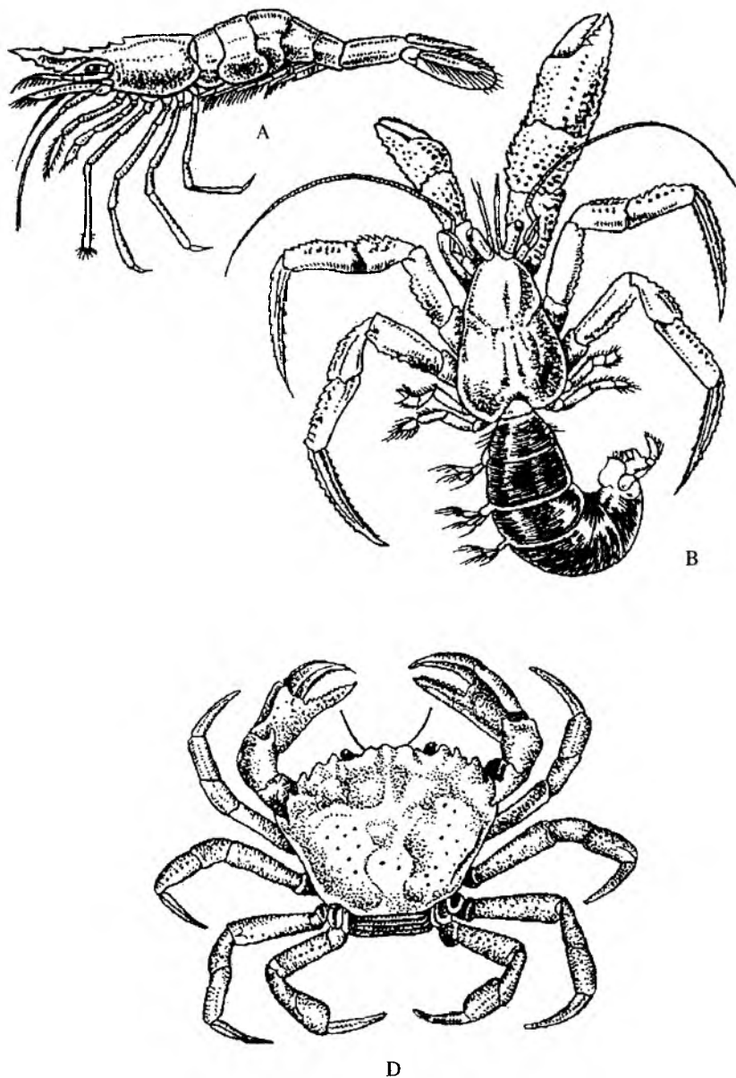
135-rasm. O'n oyoqli qisqichbaqasimonlar.
