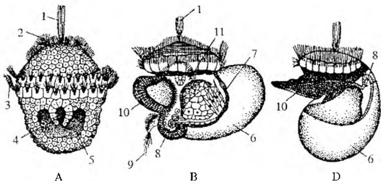
103-rasm. Qorinoyoqlilarning rivojlanishi. A – troxofora. B – yelkancha (buralishidan oldin). D – yelkancha (buralishidan so'ng): 1 – tepa toji, 2 – yuqori yarimsharlar kipriklari, 3 – prototroch, 4 – og'iz, 5 – mezodermal varaqlar, 6 – chig'anoq, 7 – ichki xalta, 8 – mantiya. 9 – orqa kipriklar, 10 – oyoq boshlang'ichi, 11 – ichak.
