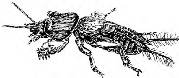
181-rasm. Buzoqboshi ( Cryllotalpa gryllotalpa ).
