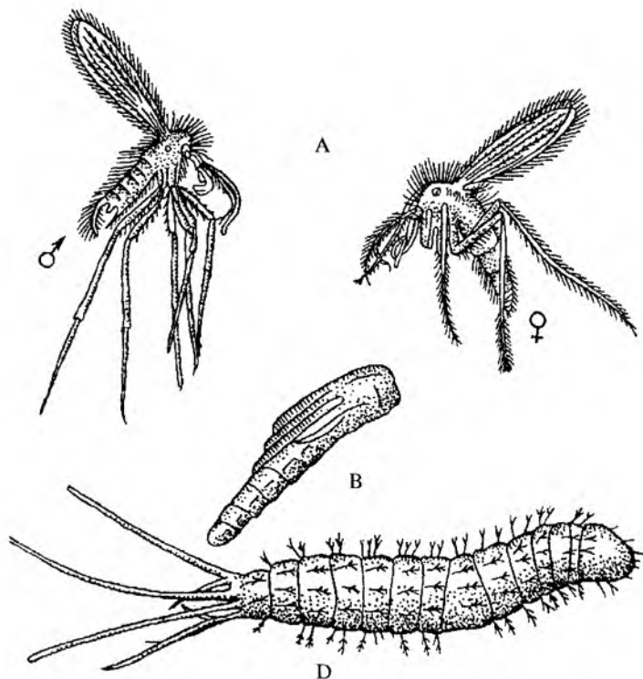
173-rasm. Iskaptopar ( Phlebotomus ).
