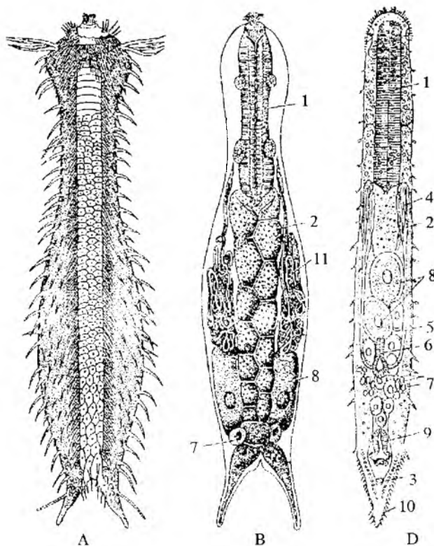
64-rasm. Qorin kipriklilar. A – chuchuk suv qorin kipriklisi Chaetonotus maximus . B – chuchuk suv qorin kipriklisi ichki tuzilishi. D – dengiz qorin kipriklisi Macrodasys bidenbrochi : 1 – qizilo'ngach, 2 – ichak, 3 – anal teshigi, 4 – urug'donlar, 5 – urug' yo'li, 6 – sirrus, 7 – tuxumdon, 8 – tuxum, 9 – kuyikish bursasi, 10 – dum, 11 – protonefridiy.
