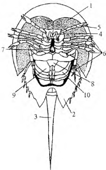
136-rasm. Qilichdum (qorin tomondan ko‘rinishi).
