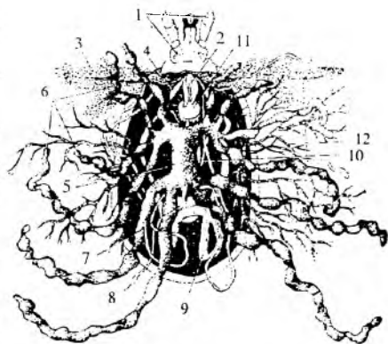
142-rasm. Iksod kanalarning ichki tuzilishi.
