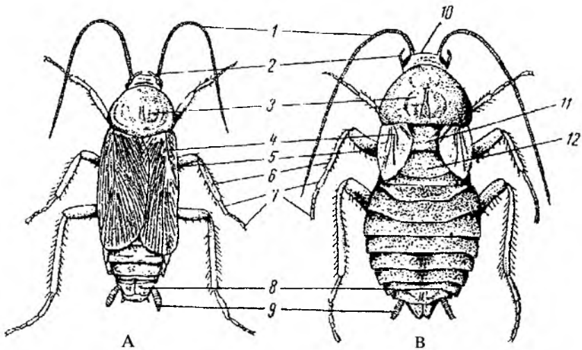
147-rasm. Qora suvarak erkagi (A) va urg'ochisi (B)ning tashqi tuzilishi. 1 – mo'ylov, 2 – jag'paypaslagichlar, 3 – oldingi ko'krak bo'g'imi, 4 – ustqanot, 5 – son, 6 – boldir, 7 – panja, 8 – qorinning uninchi bo'g'imi, 9 – serkilar, 10 – bosh, 11 – o'rta ko'krak bo'g'imi, 12 – orqa ko'krak bo'g'imi.
