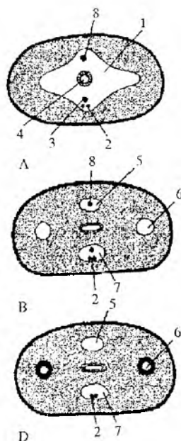
93-rasm. Zulumlarda selomning evolyutsiyasi. Qildor (A), hartumli (B), jagʻli (D) zulumlar tanasining koʻndalang kesimi: 1 – selom, 2 – qorin nerv zanjiri, 3 – qorin qon tomiri, 4 – ichak, 5 – orqa lakun, 6 – yon lakun, 7 – qorin lakun, 8 – orqa qon tomiri.
