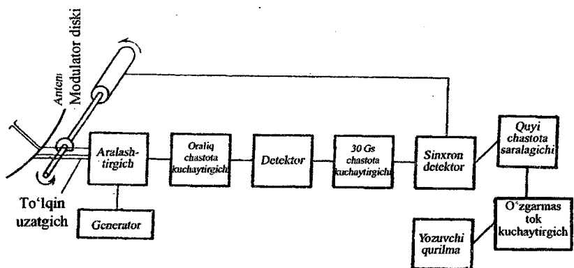
40-rasm. Modulyatsiyali radiometrning sxemasi
