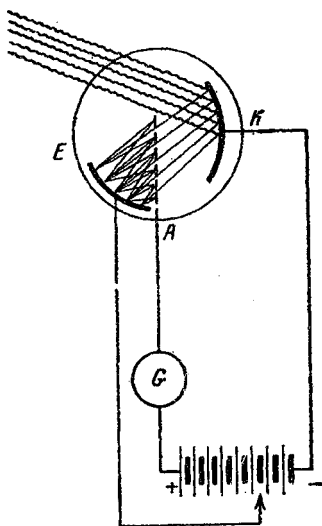
27-rasm. Bir kaskadli fotokuchaytirgich.
