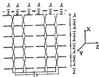
14-rasm. Koʻpdipolli antenning ulanish chizmasi.
