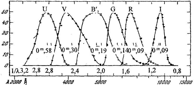
8-rasm. Kolorimetrda olti xil rangli har xil saralagichlar uchun sezgirlik chiziqlari (bir xil qo'zg'alishdagi reaksiya).
