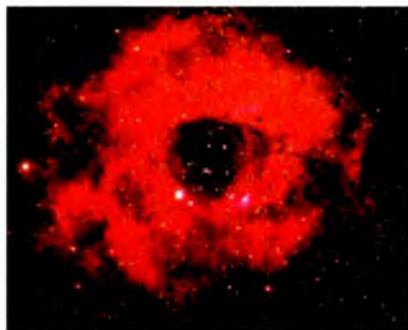
129- rasm. Yakkashox yulduz turkumidagi «Rosetka» gaz tumanligi.
