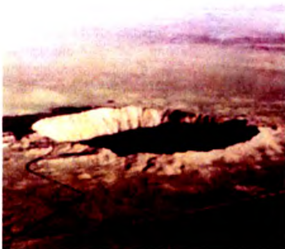
107- rasm. Arizona shtatidagi sahroga tushgan meteoritning hosil qilgan havzasi ( d = 1300 m, h = 175 m).
