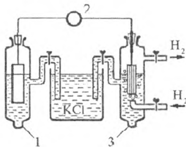
32-rasm. Noma'lum elektrodlar potentsialini o'lchash uchun ishlatiladigan elektrodlar zanjirining ko'rinishi.
