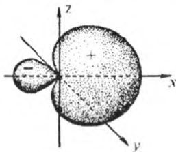
18-rasm. sp-gibrid orbitalarning alohida hosil bo'lish sxemasi.
