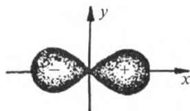
11-rasm. 2p- elektron bulutning ko'rinishi.
