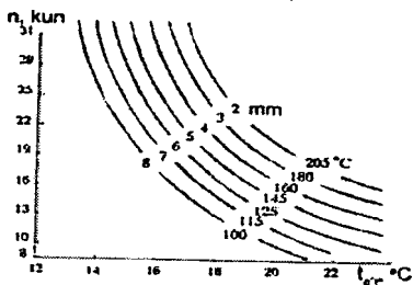
14.2-rasm. Gʻoʻza chigitini ekish-unib chiqish davri davomiyligi ( n ) ning, oʻrtacha sutkalik havo haroratiga ( t_0 , °C), samarali havo haroratlar yigʻindisi ( \Sigma t_s ) va tuproqning 0–5 sm chuqurlikdagi namligiga bogʻliqlik nomogrammasi
