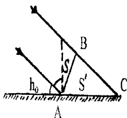
3.4-rasm. To'g'ri quyosh radiatsiyasining quyosh nurlariga tik qo'yilgan yuzadagi ( S ) va gorizontal yuzadagi ( S' ) energetik yoritilganliklari
