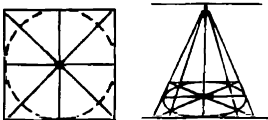
4- a rasm. Aylana perspektivasi.
