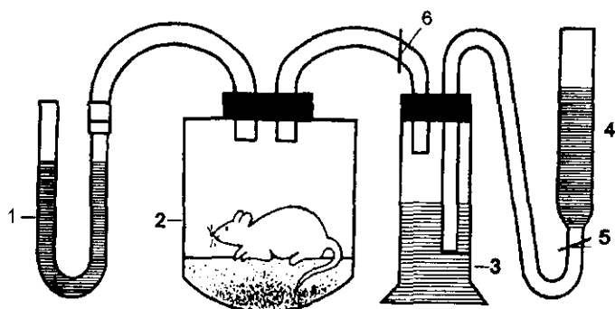
1-расм Газометрик аппаратнинг тузилиш схемаси (Колабухов қурилмаси):
