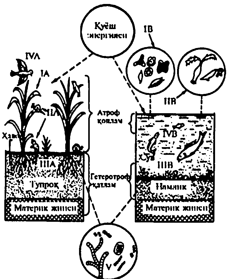
72-расм. Ўтлоқзор ва ҳовуз экосистемаларидаги трофик алоқалар
