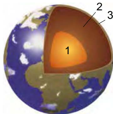
13-súwret. Jer sharınıń ishki dúzilisi.
