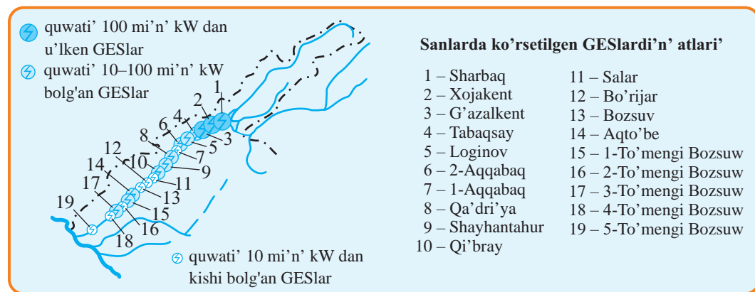
25-su'wret. Shi'rshiq-Bozsuw gidroenergetika kaskati'.
