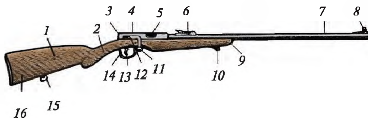
122-súwret. Kishi kalibrli miltıq (TOZ-8):
