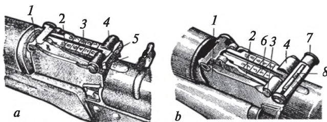
95-súwret. Nishanğa alıw úskenesi:
