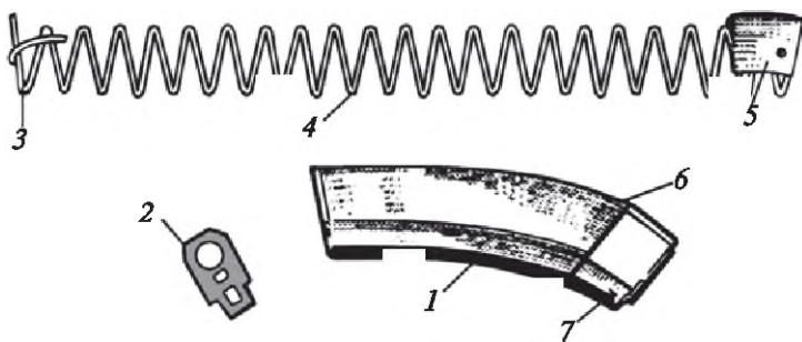
102-súwret. Magazin: 1 — korpus; 2 — qaqpáq; 3 — bekkemlewshı planka; 4 — prujına; 5 — jiberiwshi; 6 — tayanısh bōrtpesi; 7 — ilǵısh.
