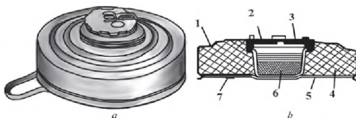
77- súwret. Tankke qarsı TM-62 M minası:
