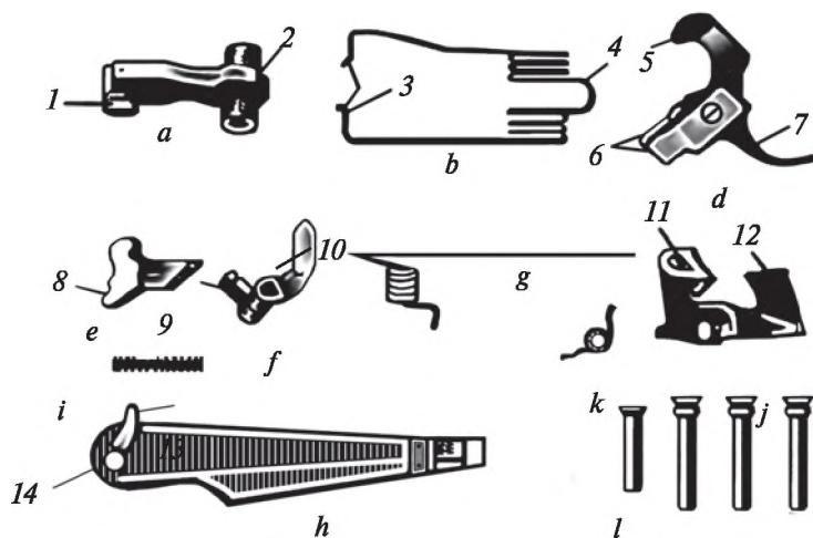
100-súwret. Soqqı beriwshi-tepki mexanizmininñ bólekleri.
