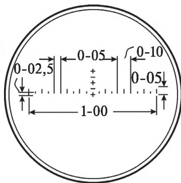
71-súwret. Dürmiyinniń múyesh ólshew shkalası.
