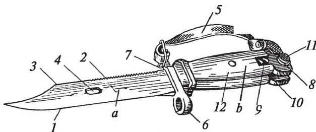
103-súwret. Nayza-pışhaq : a — tıyǵı; b — tutqası; 1 — kesiwshi jüzi; 2 — jargı; 3 — sharxlangan ushı; 4 — tesik; 5 — remen; 6 — saqıyna, 7 — remen ushın ilgish, 8 — dásteniń metall bólimi, 9 — biriktiriwshi vint, 10 — uzınsha kespe, 11 — tartqı, 12 — dáste.
