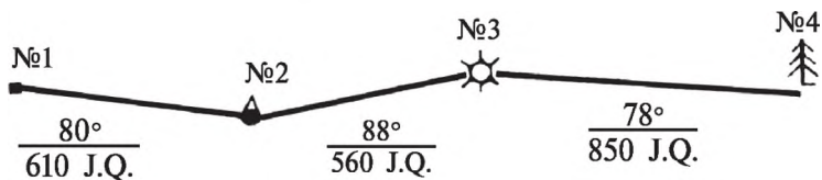
87-süwret. Azimetlar boyınsha qádemlep júriw sxeması (j.q. — jup qádem)
