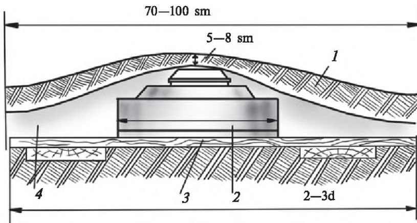
79-suwret. Tankke qarsı minanın jumsaq (ızǵar) jerde ornatılıwı.
