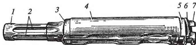
99-súwret. Gaz trubkası stvol qaplaması menen birge: 1—gaz trubkası; 2—gaz porsheni ushın bağdarlawshı qabırğalar; 3—aldıñğı biriktiriwshi; 4—stvol üsti qaplaması; 5—artqı biriktirgish; 6—börtpe; 7—jalpaq prujina.
