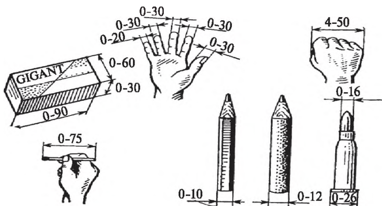
72-súwret. Qol astındaǵı predmetlerden müyeshlerdiń mırnıq shamalıqları ólshewde paydalanıw.
