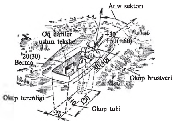
51-siwret. Avtomattan dizerlep otirip atıw ushın okop.
