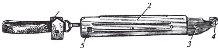
104-súwret. Qın: 1 — ildirgish, ilmekli remen hám karabin menen birgelikte; 2 — plassmassalı qabı; 3 — oq-bórtpe; 4 — tayanshı; 5 — jalpaq prujına biriktiriwshi.
