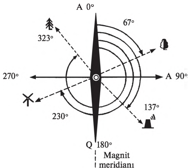
86-süwret. Magnit azimutları.
