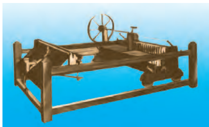
«Jenni» mehaniki ýüp egirýän maşyny.
